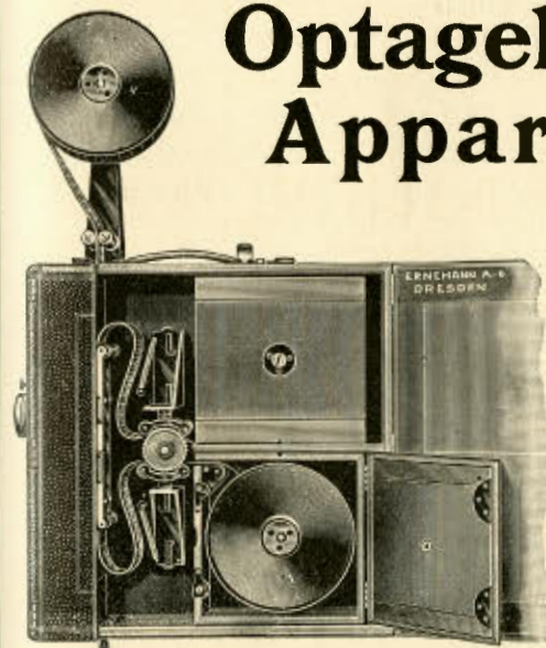
Model A med Kopier Mekanisme
