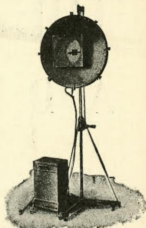
»Jupiter-Soleffektlampe« med Frembygning uden Matskive
